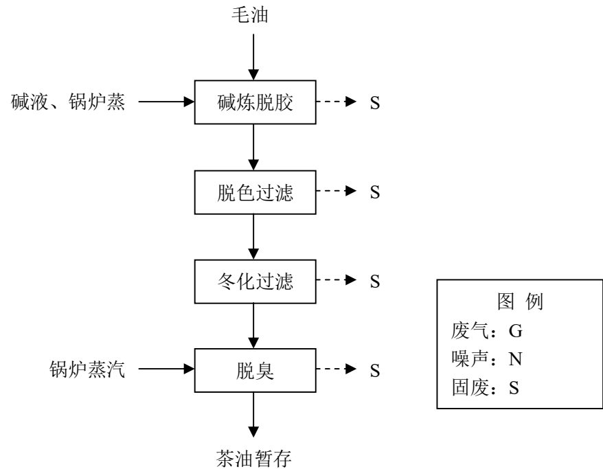
图 2.2-2 茶油精炼加工工艺及产排污流程
