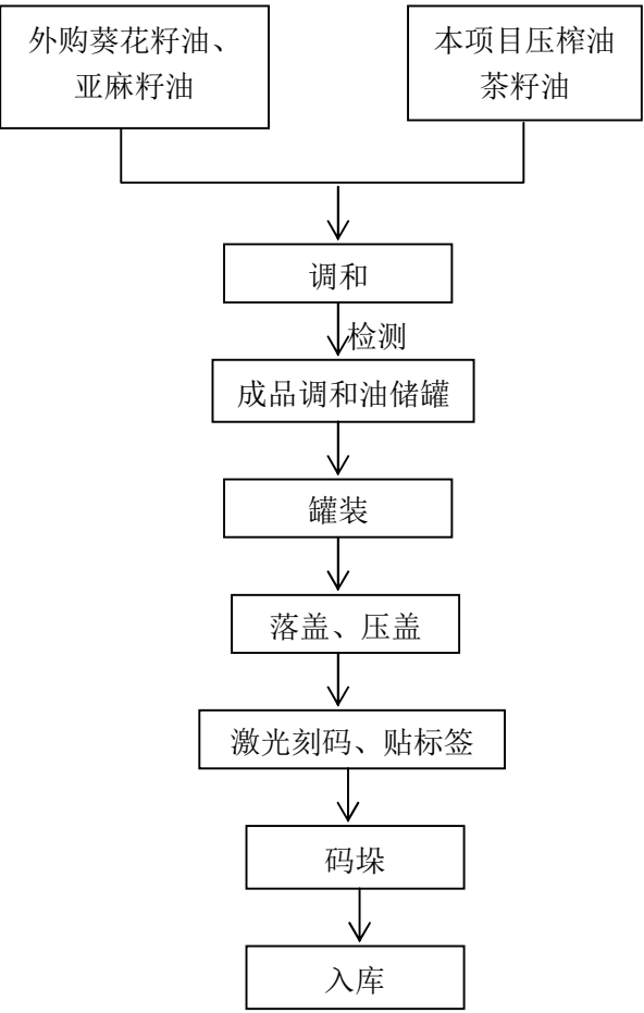
附图 2.2-3 调和及灌装工艺流程图
