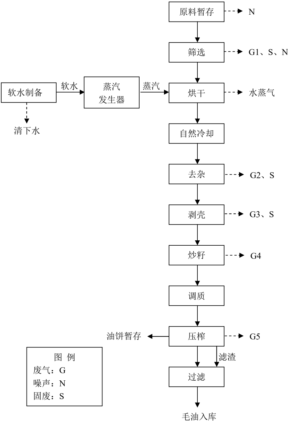
图 2.2-1 毛油加工工艺及产排污流程
