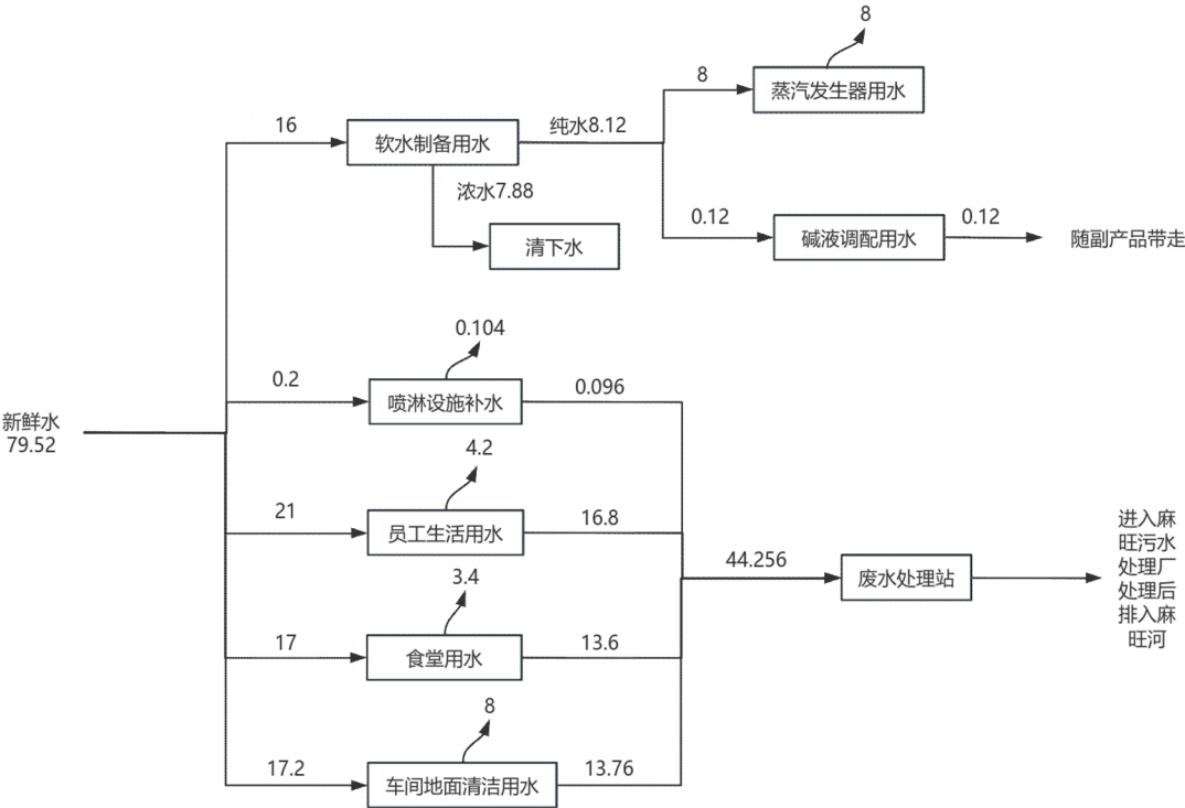
图 2.1-2 项目水平衡图 单位：m³/d
