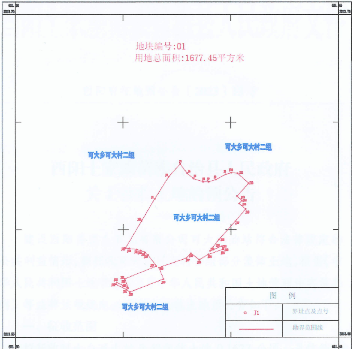
西阳县宜人石化有限公司可大加油站勘测定界图
